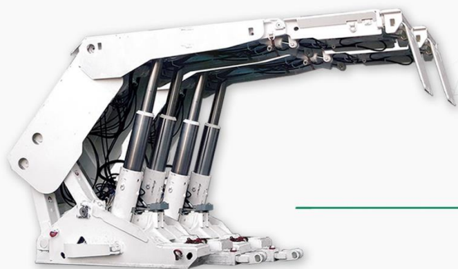
工作面液压支架系统
