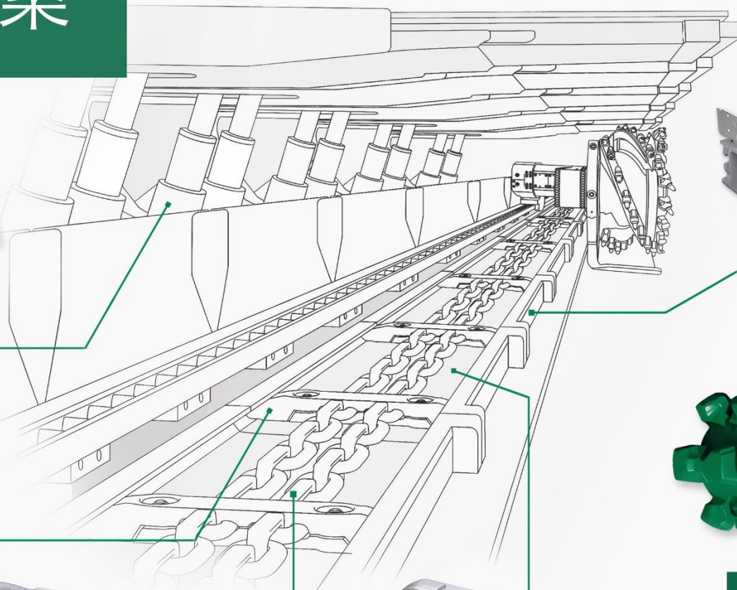
输送机槽板
