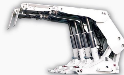
液压支架
