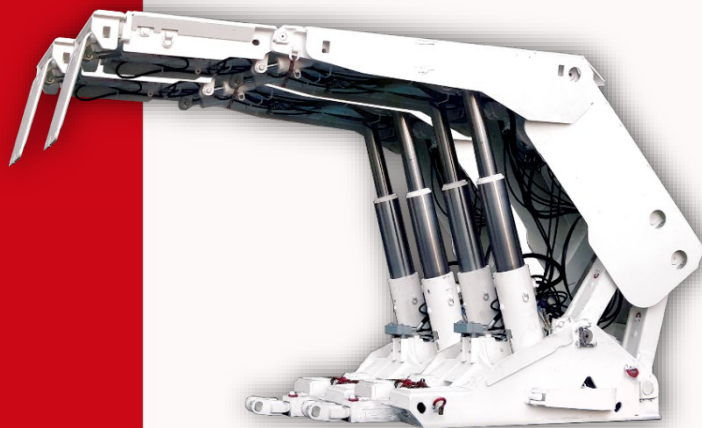
OBUDOWY ZMECHANIZOWANE
